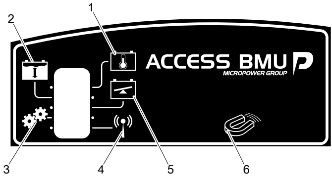
Fig. 2 Access™ BMU
